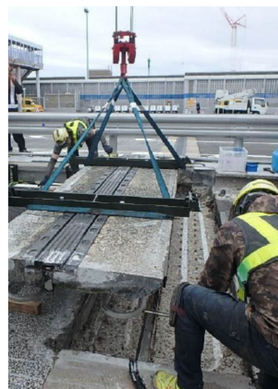
ブロック状の一括吊り上げ
