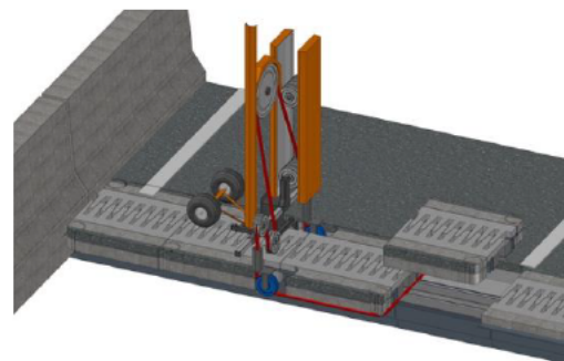
SJS 工法(水平切断機械)
