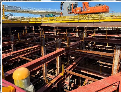
①換気所 掘削工
