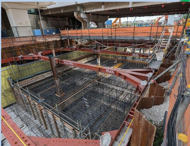
③擁壁部の鉄筋・型枠組立
