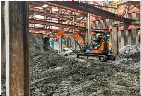
④トンネル部の地盤掘削
