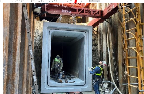
⑥下水幹線敷設工
