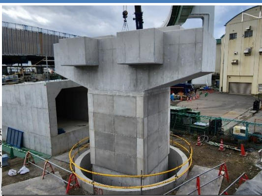
②橋脚本体の構築
