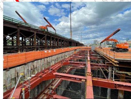
⑥ 換気所掘削
