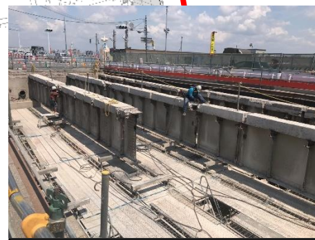
⑦ 既設橋梁撤去
