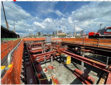
⑦ 換気所掘削
