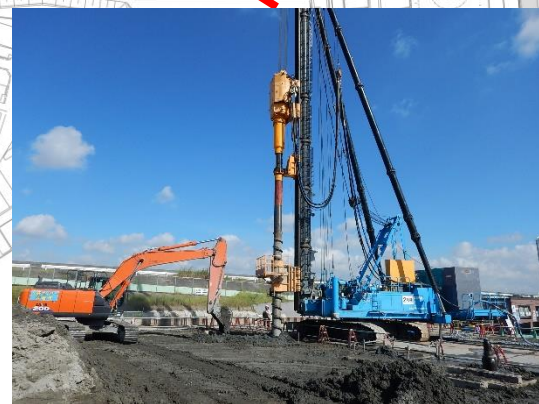
地盤改良
