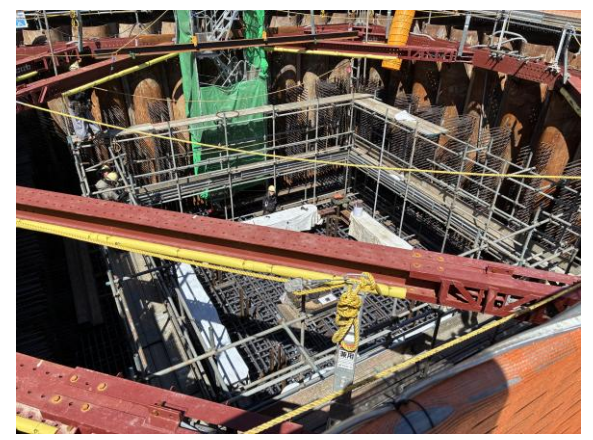
【3】橋脚工事(PPE-6)において、アンカーフレーム設置中。
