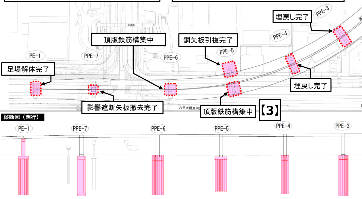
【3】橋脚工事(PPE-5L)において、頂版鉄筋構築中。
