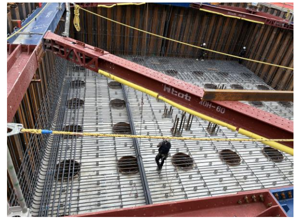
【3】橋脚工事(PPE-5L)において、頂版鉄筋構築中。
