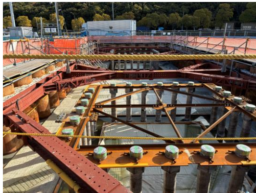
【3】橋脚工事(PPE-4)において、頂版コンクリート 打設完了
