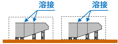
PPE-1 鋼製柱地組溶接中
