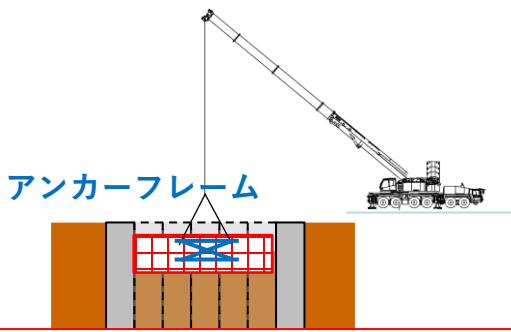
PPE-2 アンカーボルト設置完了
