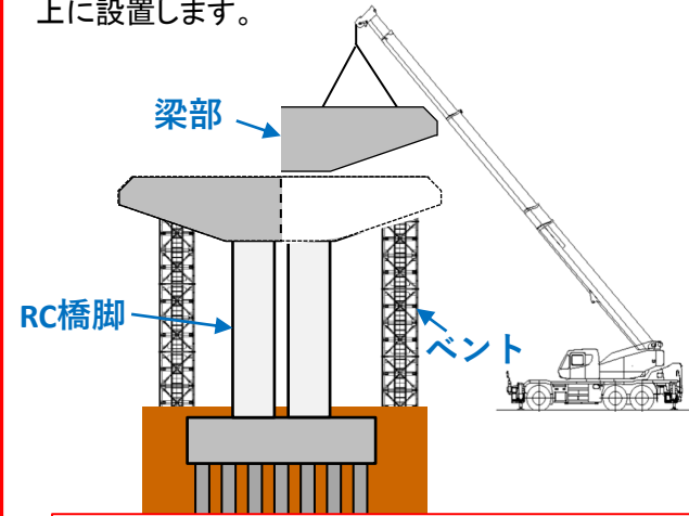
PE-1 鋼製梁架設(足場設備解体)完了
