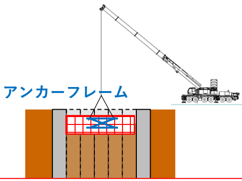
PPE-4 アンカーフレーム設置完了
