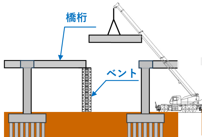
③橋桁の架設
