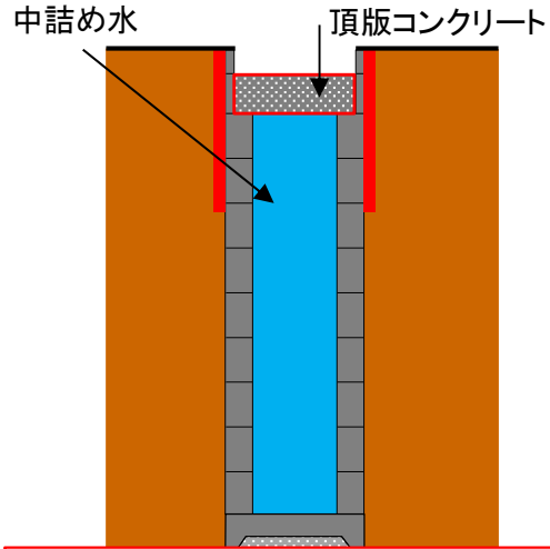
⑦中詰め水の注水、 頂版コンクリート打設
