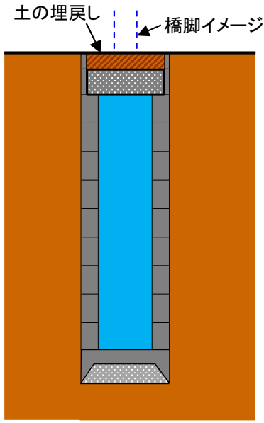
⑧影響遮断矢板撤去
