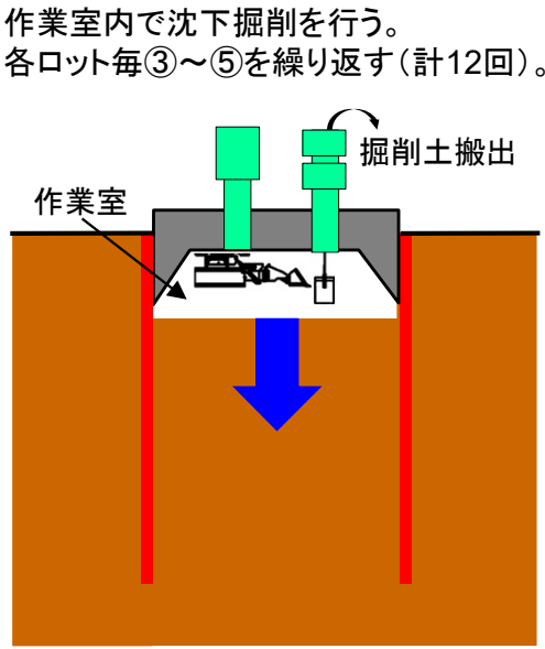
⑤沈下掘削
