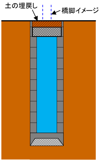
⑧影響遮断矢板撤去
