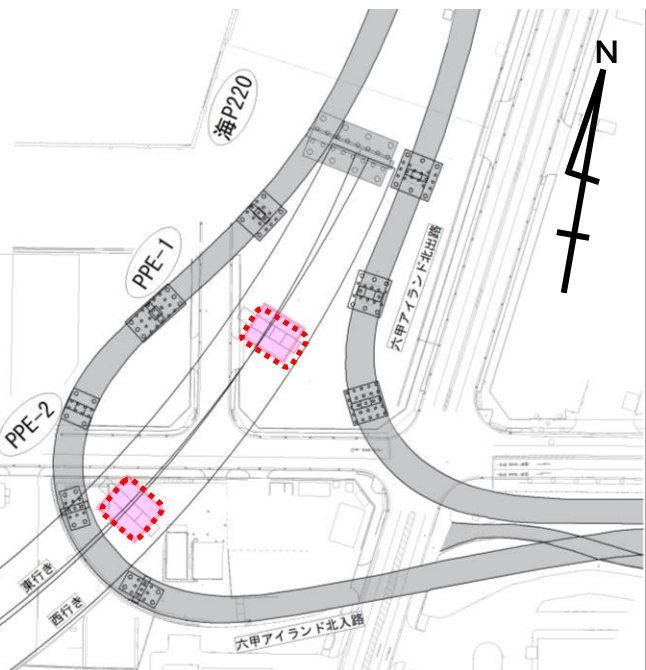
写真③ PPE-1 頂版コンクリート打設完了 PPE-2 鋼管矢板打込完了
