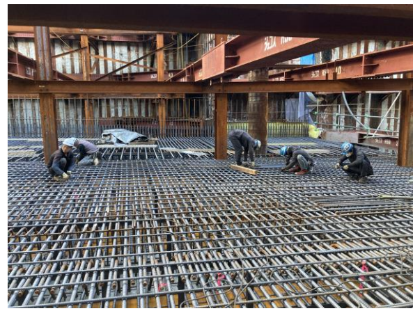
【2】施工区間④ 10-1ブロック 中床版上筋組立状況
