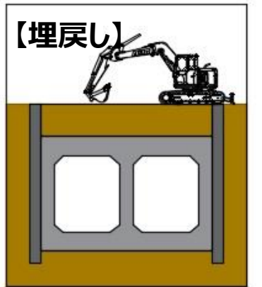
【埋戻し】 (8) 切梁を外し、 埋め戻し。
