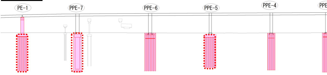
縦断図 (西行)
