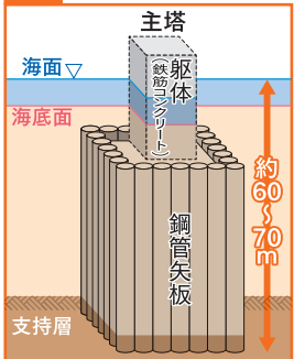
図A 主塔基礎イメージ図
