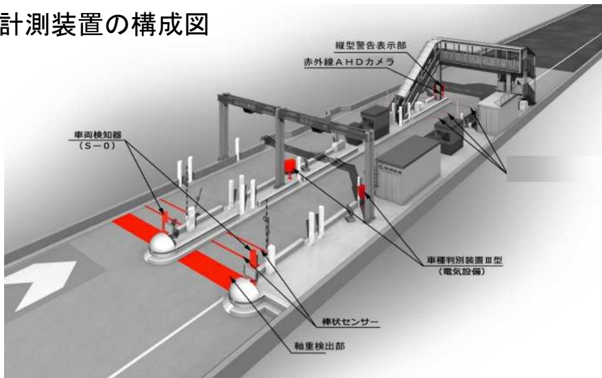
重量検出装置(施工後)
