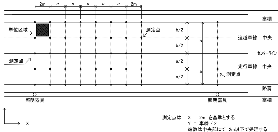
図 1.3.1-1 照度測定方法
