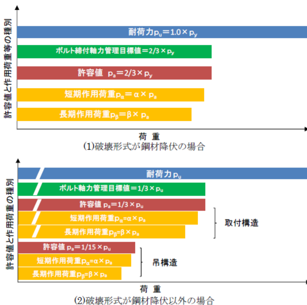
別図 引張試験における管理目標値
