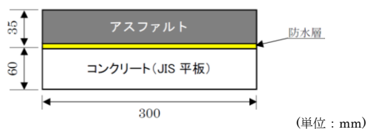
図 試験体
